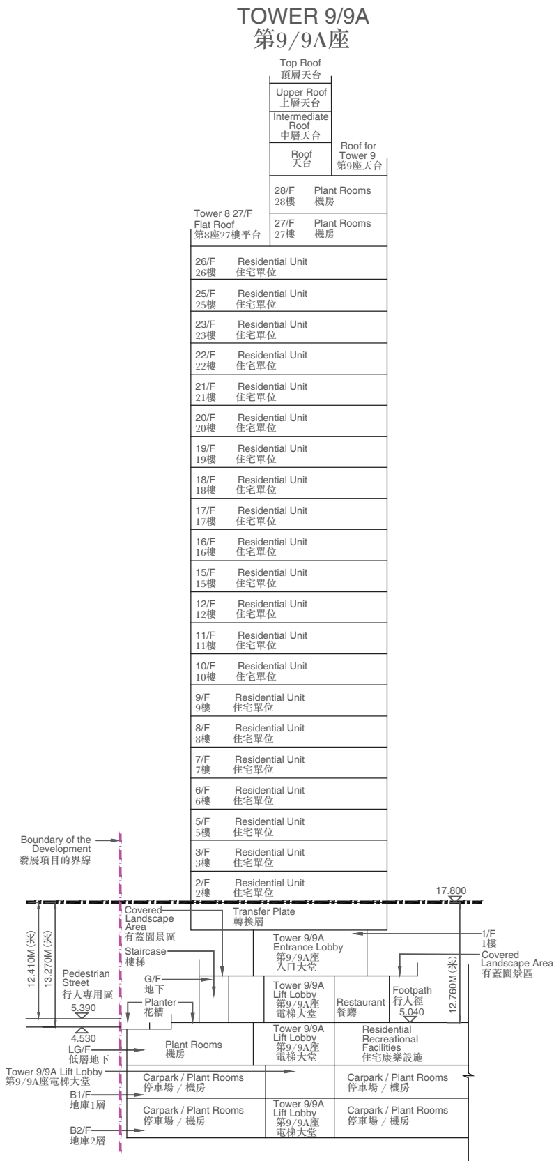
CROSS-SECTION PLAN C-C 橫截面圖 C-C
